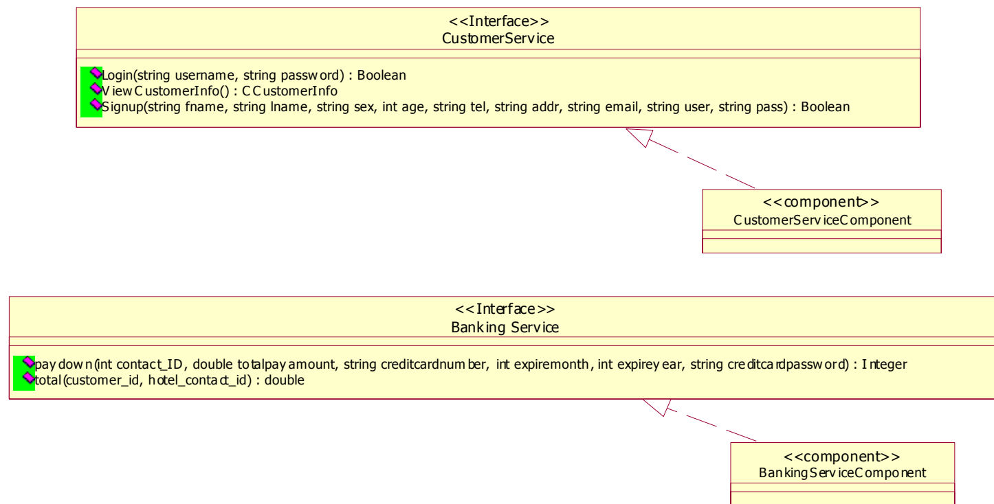
รูปที่ 8-34 class diagram ระบบโรงแรม (หน้าที่ 1)
